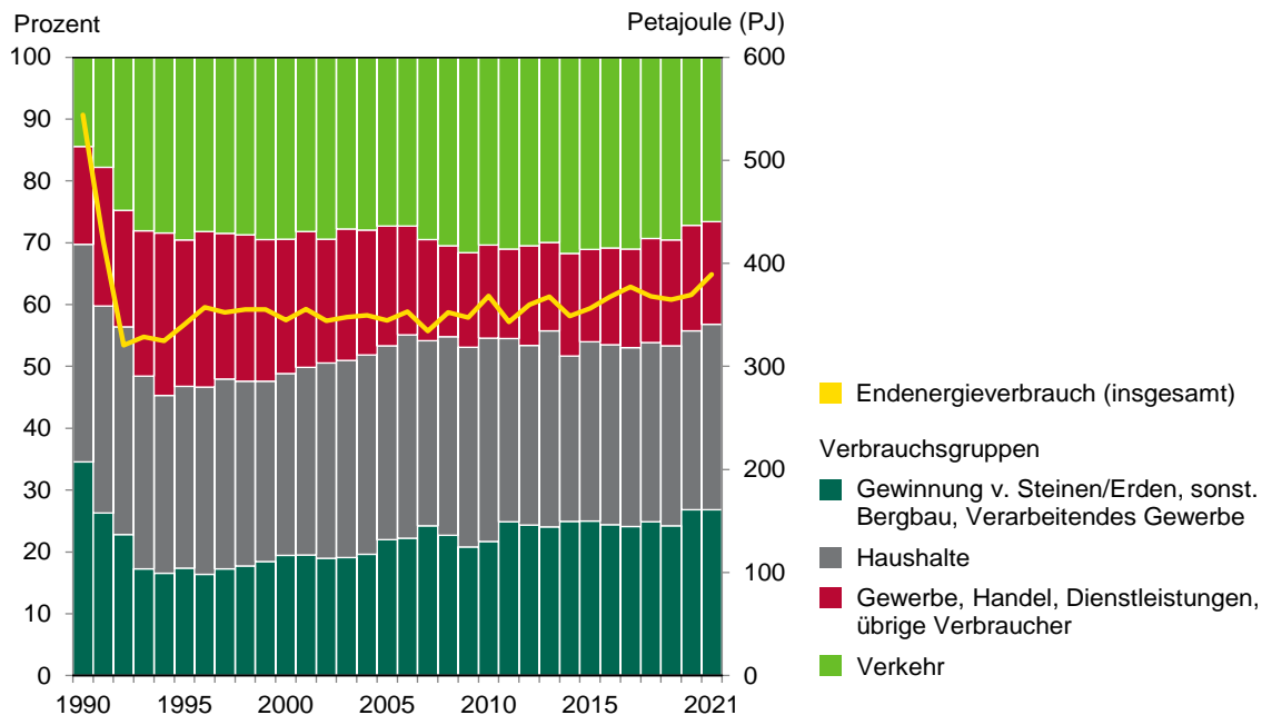
Abb. 2 Endenergieverbrauch nach Verbrauchsgruppen in Sachsen 1990 bis 2021
